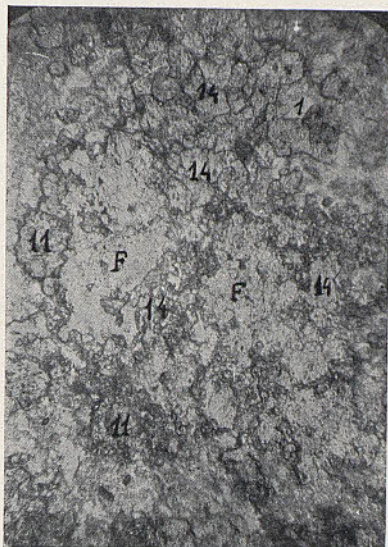
FIG. 2. Diopsidita del Moli Vell. L. ord. 20 d.; 11, granate; 14, diopsido; F, masa filítica; 1, cuarzo
