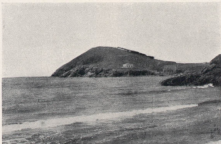
FIG. 2. El Cap Gros desde La Fosca ; a la derecha se ve parte de La Negra
