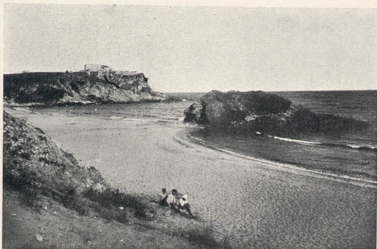
FIG. 2. Cala de La Fosca, lado NE. y Centro; en éste la roca llamada « La Negra »
