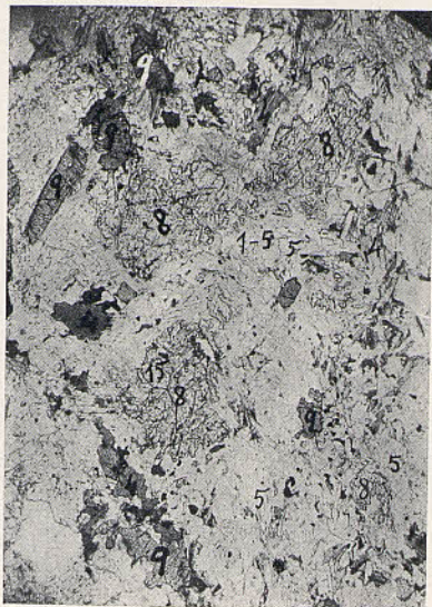
FIG. 1. Neis andalucítico del lado NE. de La Fosca. L. ord. 20 d. ; 4, biotita ; 5, cuarzo ; 8, andalucita ; 9, turmalina ; 15, apatito ; 1-5, pasta de feldespatu y cuarzo
