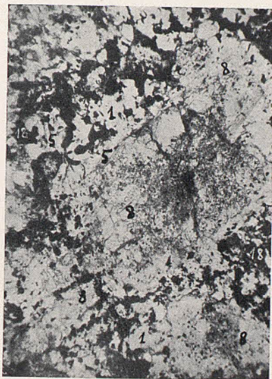
FIG. 4. Pizarra maclífera de La Negra. L. ord. 15 d. ; 1, cuarzo ; 5, moscovita ; 8, quíastolita ; 18, carbón
