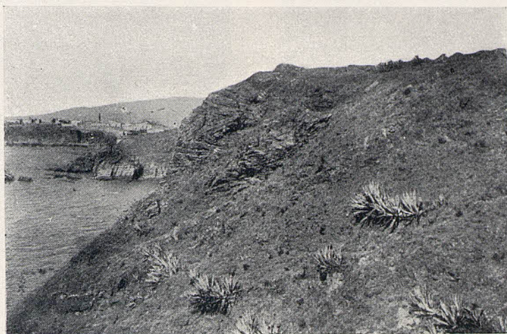
FIG. 1. Calizas marmorizadas devónicas replegadas del lado Sur del Cap Gros
